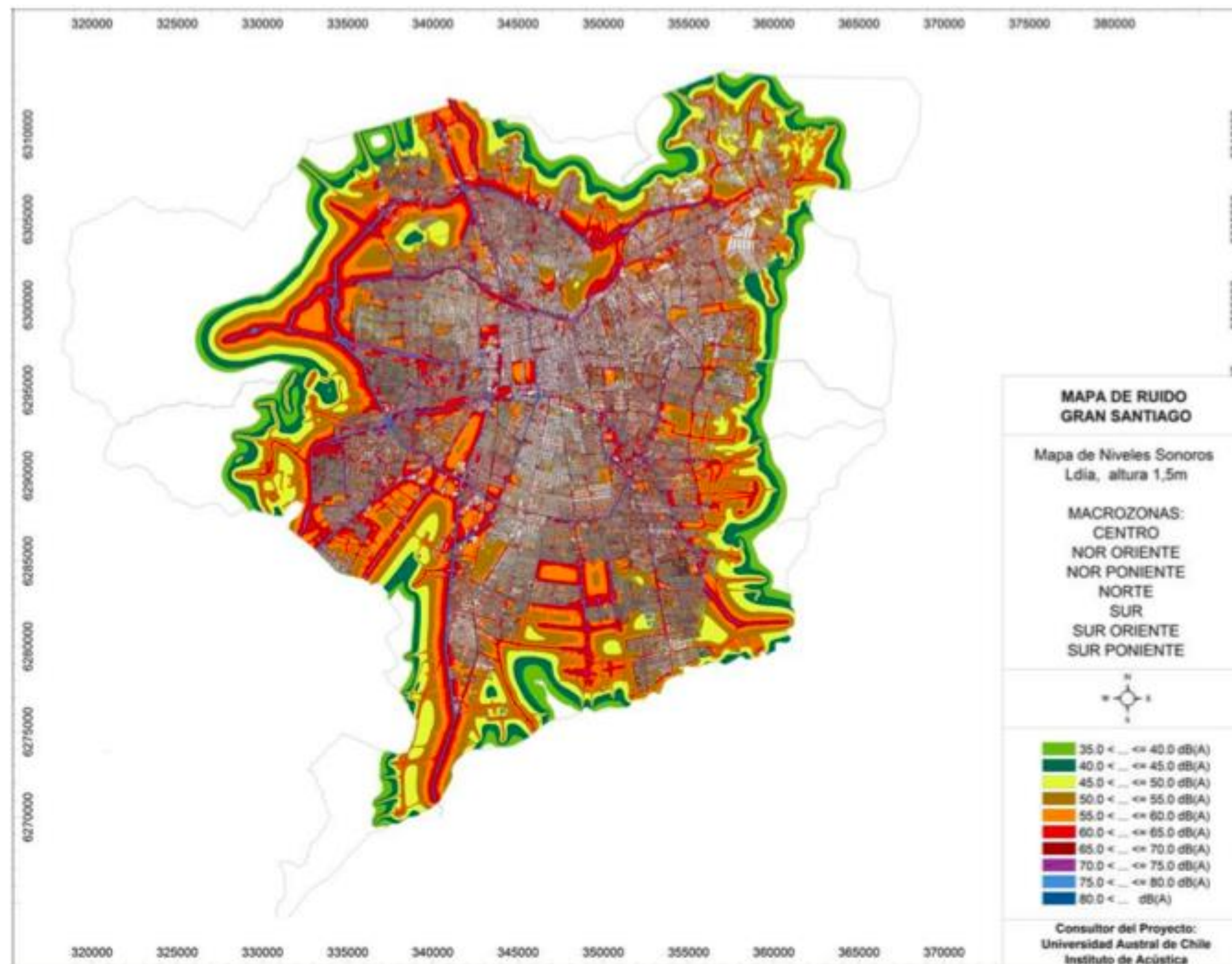
Figura 3.2.1. Mapa de Ruido del Gran Santiago 2011 [19].
